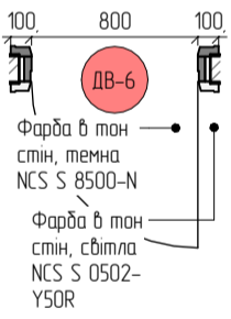
Скляна перегородка розсувна
