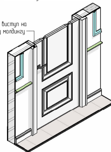
Деталь стику лиштви з молдингом
