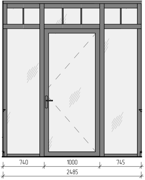
Двері вхідні
