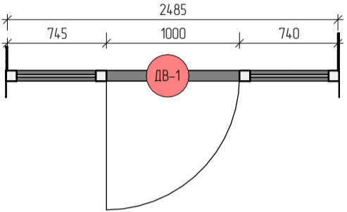
Двері з ліштвою
