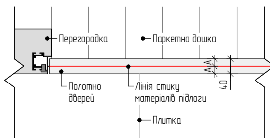
Вузел стику різних матеріалів підлоги
