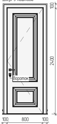
Двері з лиштвою
