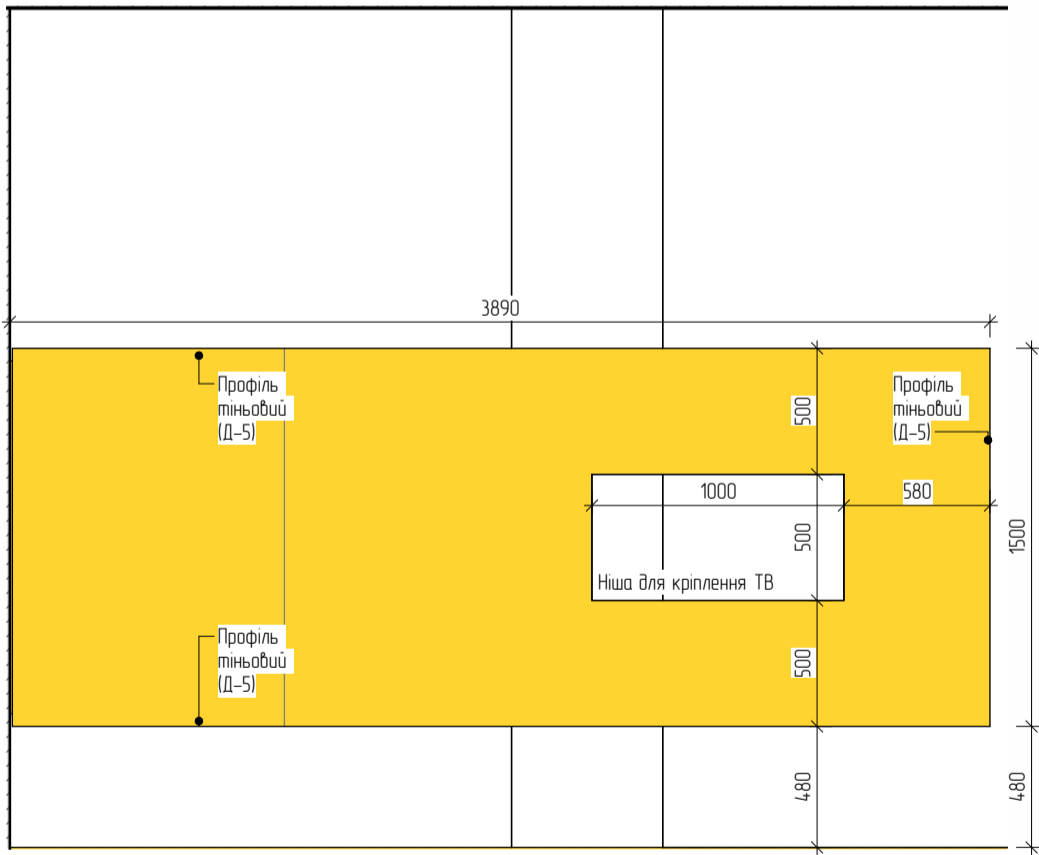
Вузел 13
