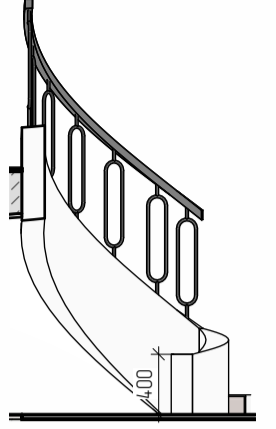
Розріз 9.3
