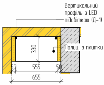
Вузел 2
