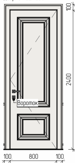
Двері з лиштвою
