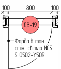
Двері з лиштвою
