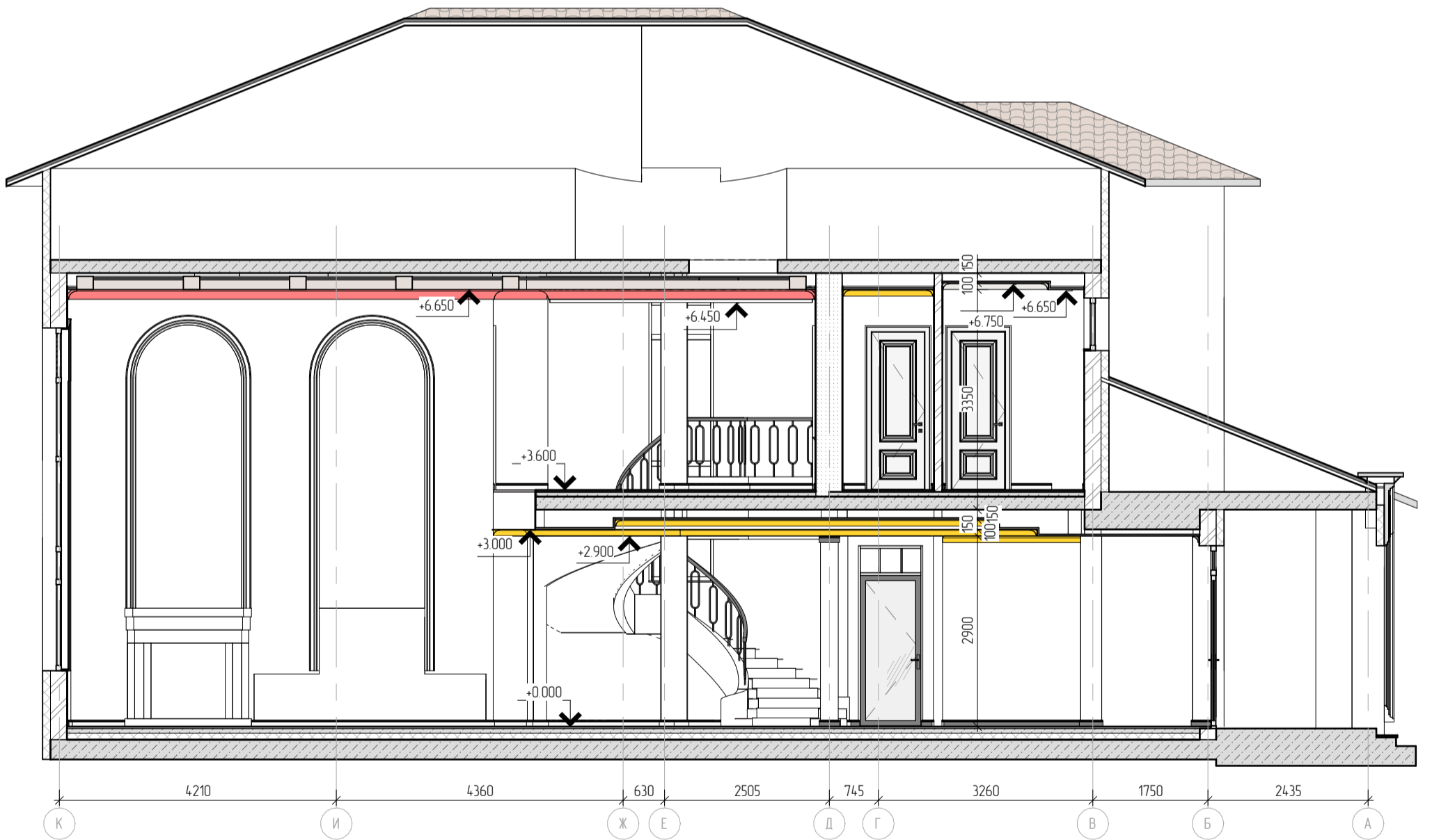
Розріз підлоги 2-2
