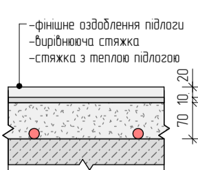
Розріз підлоги 3-3
