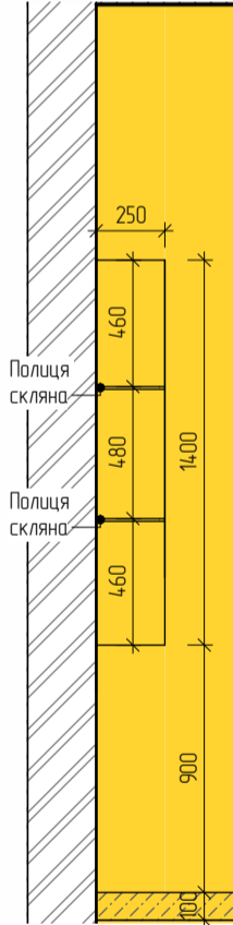
Вузел 2
