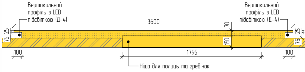
Вузел 12
