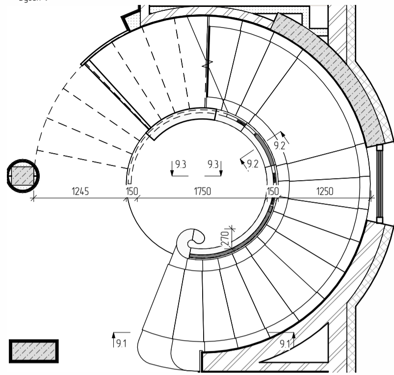
Вузел 9
