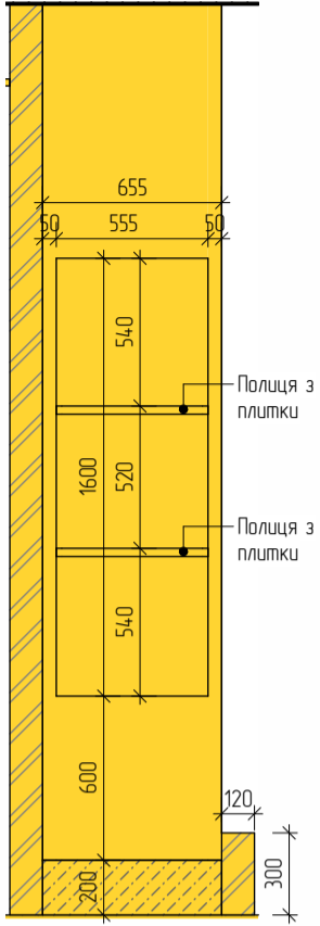
Вузел 1
