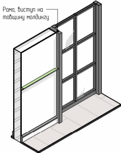
Деталь 1
