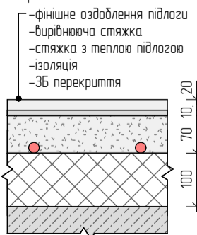
Розріз підлоги 1-1
