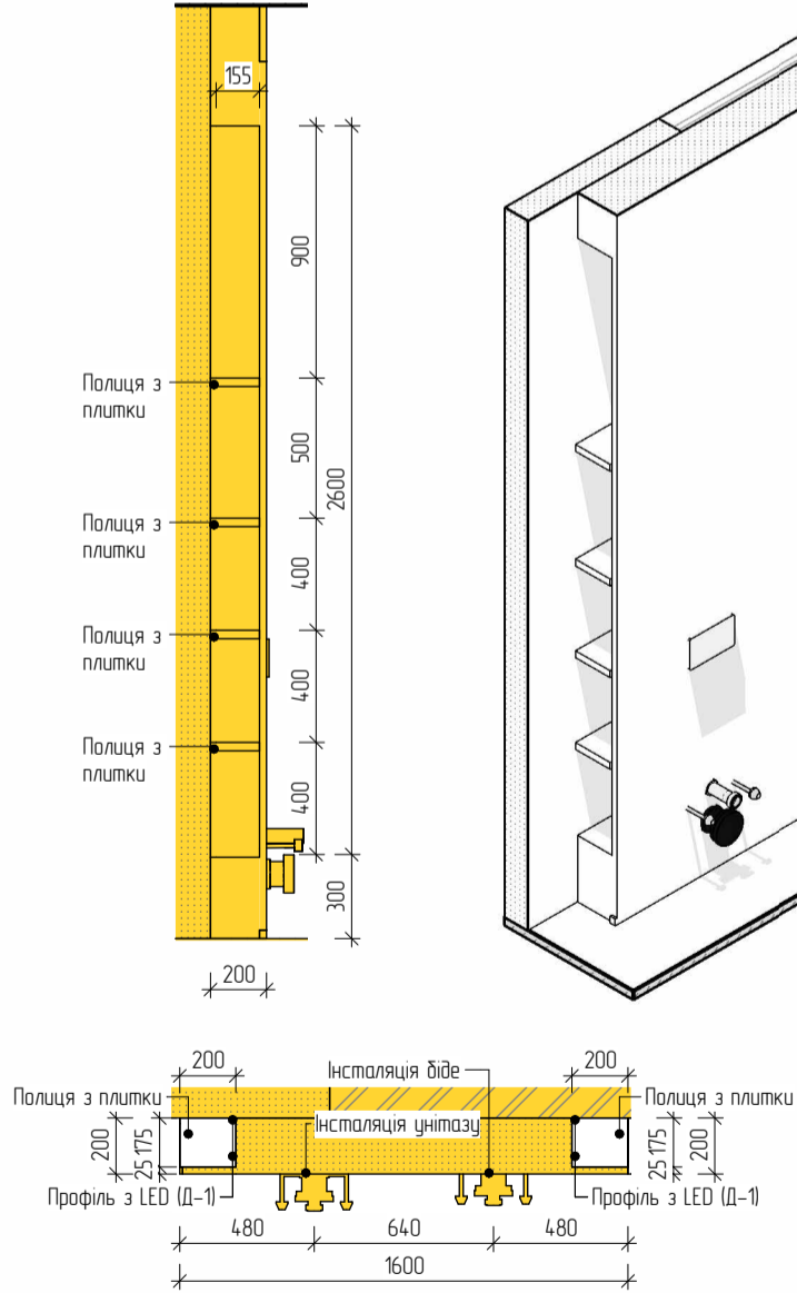
Вузел 4
