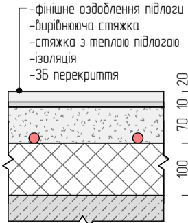
Розріз підлоги 1-1
