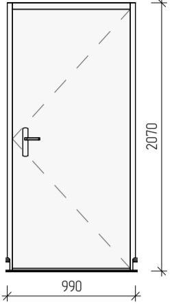
Двері вхідні
