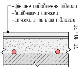
Розріз підлоги 3-3
