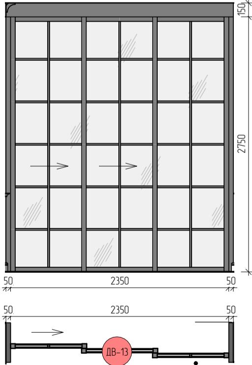
Скляна перегородка розсувна
