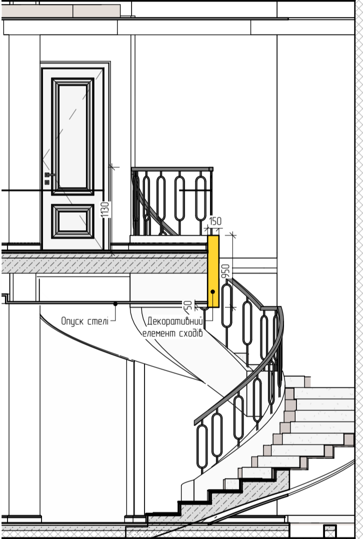
Розріз 9.1
