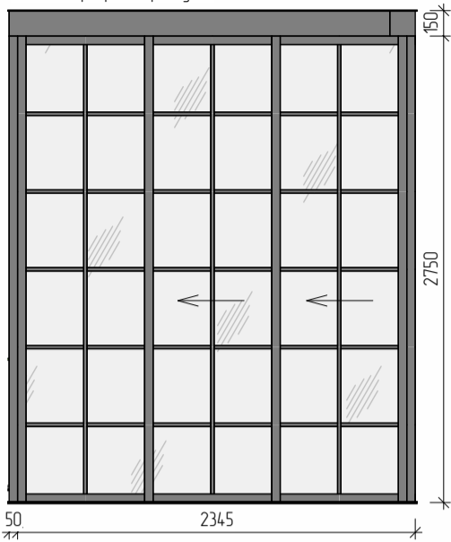
Скляна перегородка розсувна
