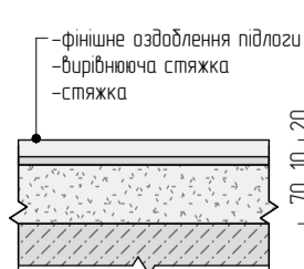
Розріз підлоги 2-2
