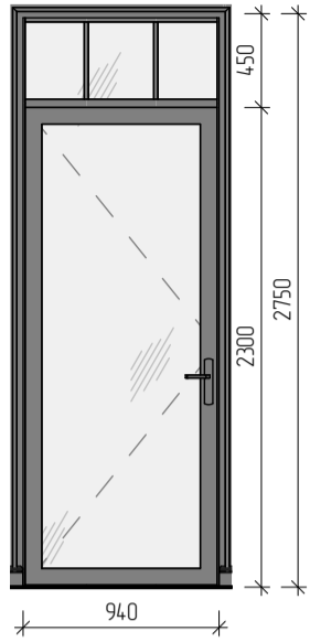
Двері вхідні
