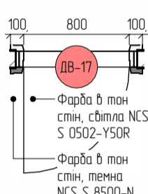
Двері з лиштвою
