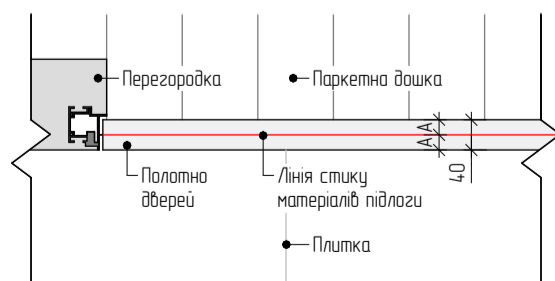
Вузол стику різних матеріалів підлоги
